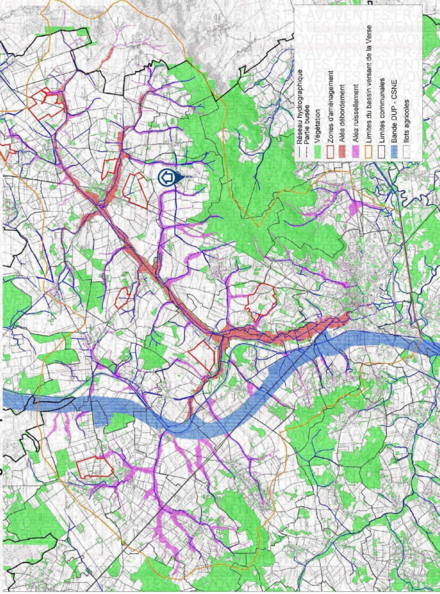
Carte du réseau hydrographique du bassin versant de la Verse et zones d'aménagement pouvant lutter contre le ruissellement
